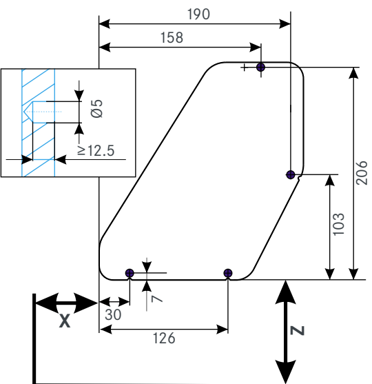
Borebillede til eurosruer
