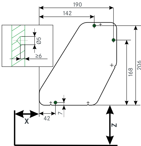
Borebillede til positioneringstapper
